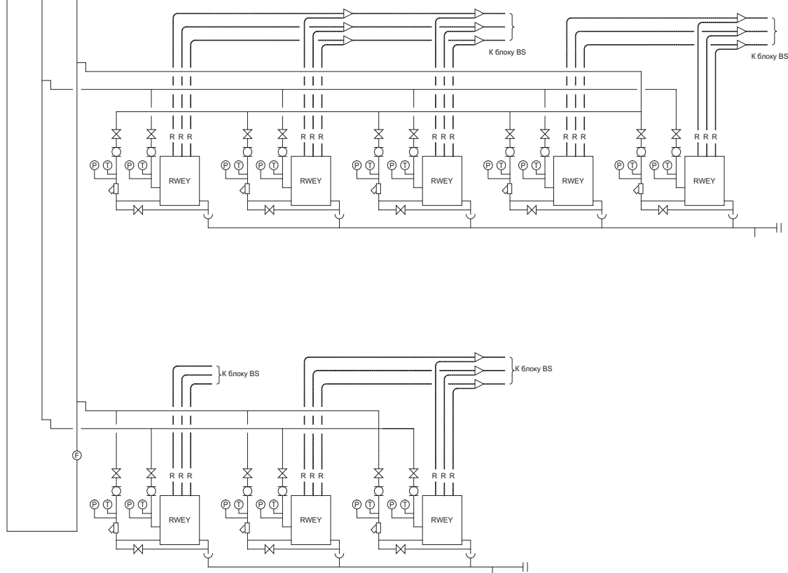
Регулирование T1
