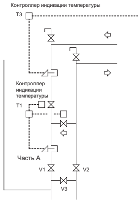
Типовая модификация для Части А (трехходовой клапан → двухходовой клапан)
