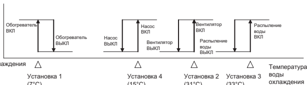
Регулирование T3
