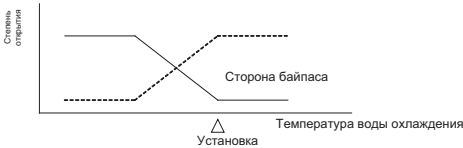
Регулирование T2
