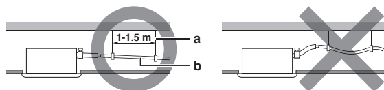
Fig. 4.18: Установка дренажного трубопровода
