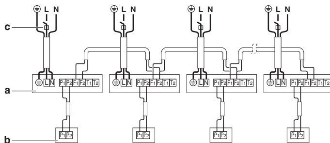
Fig. 4.15: 1 пульт ДУ для 1 внутреннего агрегата
