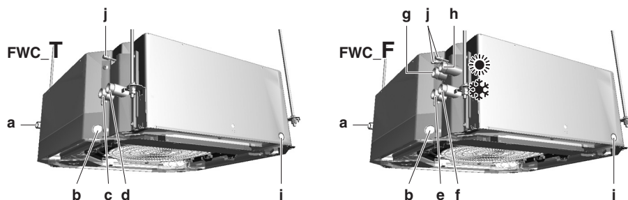
Fig. 4.10: Соединение трубопроводов воды
