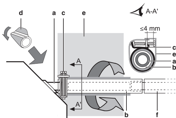
Fig. 4.22: Обертывание уплотнительной подушкой
