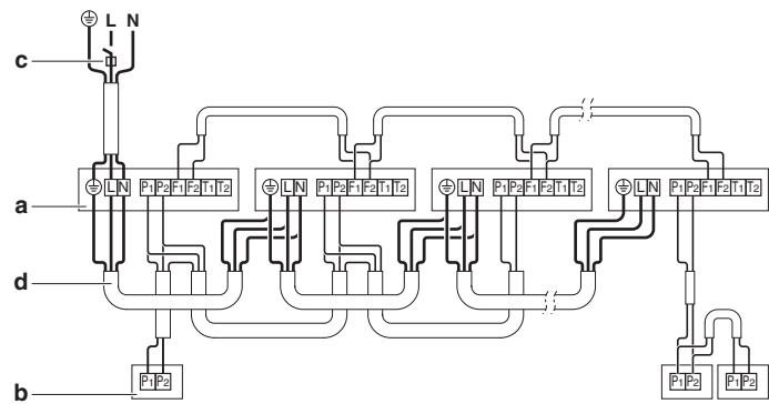
Fig. 4.16: Групповое управление или использование с 2 пультами ДУ
