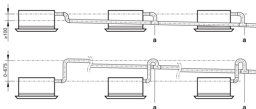
Fig. 4.20: Объединение нескольких дренажных труб
