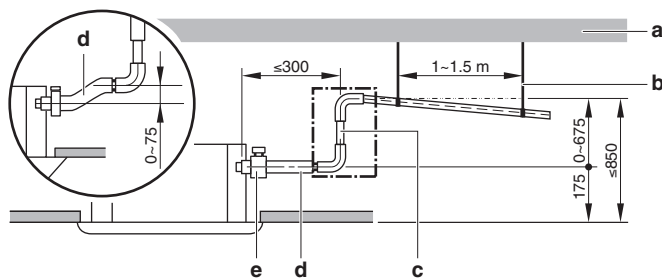
Fig. 4.19: Как работать с дренажным трубопроводом
