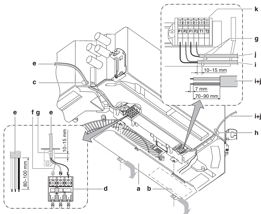
Fig. 4.17: Как подсоединить электропроводку
