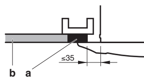
Fig. 4.3: Слишком большое потолочное пространство
