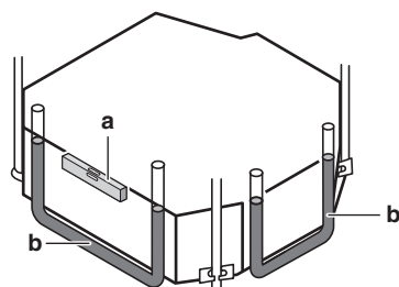
Fig. 4.9: Проверьте выравнивание агрегата
