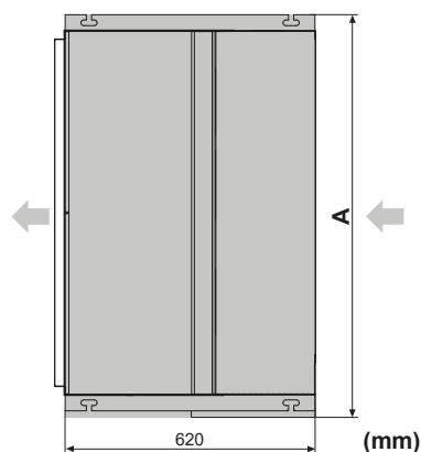
16-1 Размеры отверстия в подвесном потолке (А)
