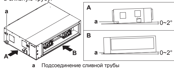
a Подсоединение сливной трубы
