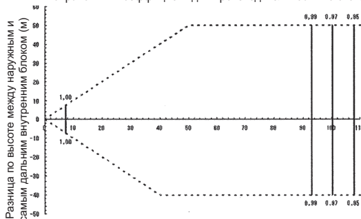
Поправочный коэффициент для производительности по отоплению
