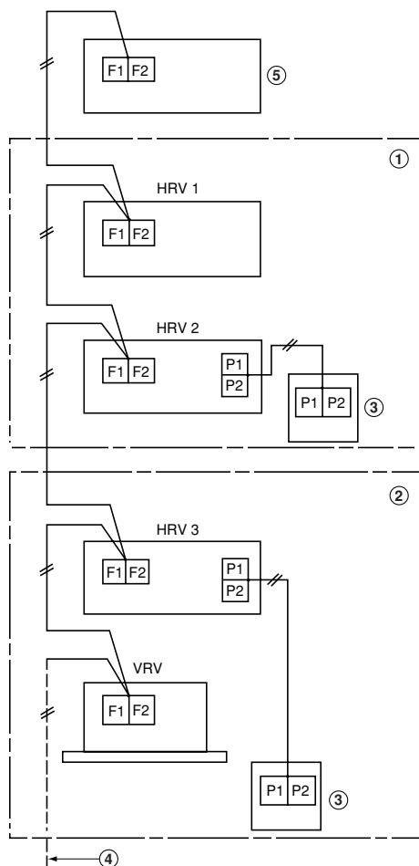
1 Зона 1 2 Зона 2 3 Дистанционный контроллер для HRV 4 Длина соединительной линии может быть увеличена максимум до 1000 м. 5 Централизованный контроллер (DCS302B61)
